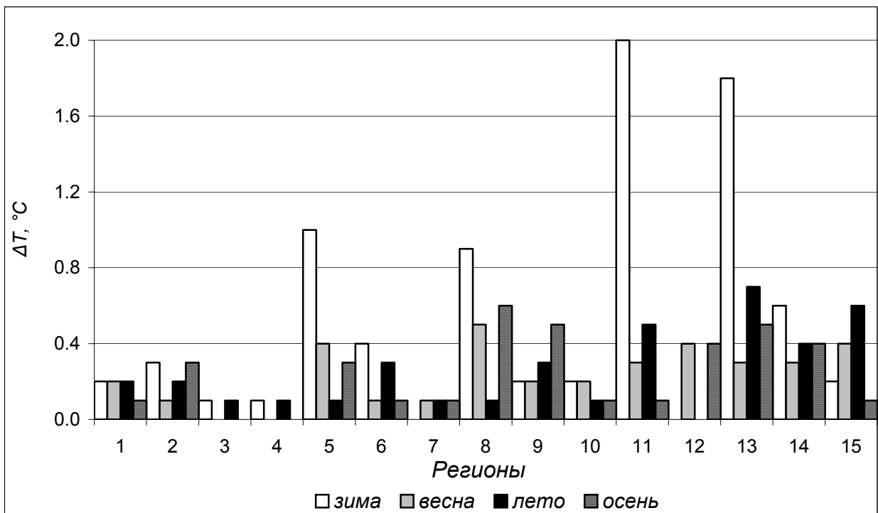
Рис. 3. Абсолютные разности сезонных региональных трендов температуры, рассчитанных по данным объединенного архива за период 1976-2009 методом простого арифметического осреднения и весового осреднения с использованием полигонов Вороного-Тиссена.
