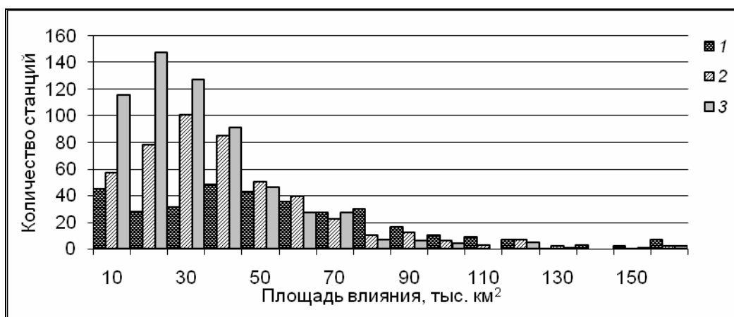
Рис. 2. Гистограммы распределения полигонов Вороного-Тиссена метеостанций (площадей влияния) для различных архивов. Расчет для станций, имеющих не более 20% пропусков наблюдений в период 1976-2008. 1 - архив ИГКЭ (455 станций), 2 - архив ВНИИГМИ-МЦД (518 станций), 3 - объединенный архив (744 станции).
