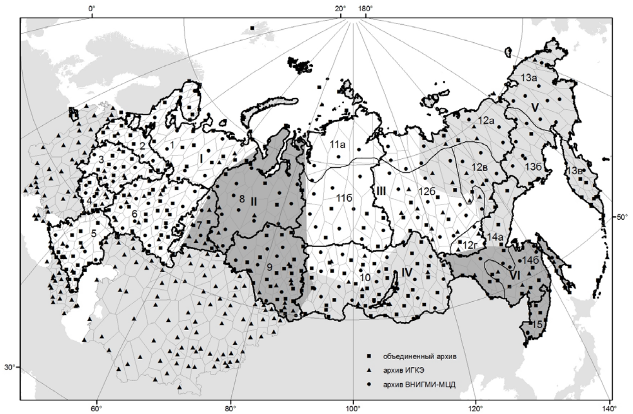
Рис. 1. Варианты дискретизации территории России с выделением различного числа регионов. Фоновой заливкой выделены 6 регионов (обозначены римскими цифрами); сплошные контуры – 15 регионов (обозначены арабскими цифрами); тонкими линиями обозначено деление, дополняющее число регионов до 22 (обозначены буквенными индексами после номера региона). Тонкими серыми линиями показаны полигоны Вороного-Тиссона для станций объединенного архива.
